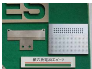
細穴放電パーツ
